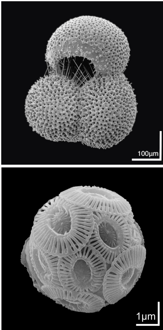
Abb. 4.6-1: Elektronenmikroskopische Aufnahmen der Coccolithophoridenart Emiliana huxleyi (B) und der Foraminiferenart Globigerinoides ruber . E. huxleyi gehört zum Phytoplankton und lebt somit an der Meeresoberfläche, wo genug Licht für Photosynthese vorhanden ist. Wenn die Kalkalge die für sie typischen Blüten bildet, kann man dies sogar durch eine milchige Färbung des Meerwassers vom Weltall aus sehen kann. G. ruber gehört zum Zooplankton und lebt an der Oberfläche, wo es anderes Zooplankton frisst. Coccolithophoriden und Foraminiferen sind die produktivsten Kalkbildner unseres Planeten. Ihre kalkigen Überbleibsel, die über lange Zeit auf den Meeresgrund gesunken und dort akkumuliert sind, finden wir heute in Form von mächtigen Kalkformationen wieder. Dazu gehören zum Beispiel die Kreidefelsen der englischen Südküste in Dover. Elektronenmikroskopische Aufnahmen wurden am Institut für Geowissenschaften der Universität Kiel angefertigt (Fotos: L. T. Bach, M. Regenberg & K. Nachtigall).
