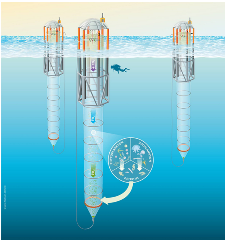
Abb. 4.6-2: Schematische Darstellung der pelagischen Mesokosmenanlage KOSMOS (Kiel Off-Shore Mesocosms for Ocean Simulations), die am GEOMAR Helmholtz-Zentrum für Ozeanforschung Kiel entwickelt wurden (RIEBESELL et al. 2013). Ein 8 m langes Schwimmtor trägt einen 25 m langen zylindrischen Sack aus lichtdurchlässiger Kunststoffolie. In diesem Sack werden ca. 50 m 3 Meerwasser inklusive der darin natürlich vorkommenden Planktongemeinschaft eingeschlossen. In einem Experiment kommen bis zu zehn solcher Säcke zum Einsatz, welche dem experimentellen Design entsprechend unterschiedlich manipuliert werden können. Für Experimente zur Ozeanversauerung wird das Karbonatsystem des eingeschlossenen Wassers durch Zugabe von \text{CO}_2 -gesättigtem Seewasser so eingestellt, dass es die für die Zukunft prognostizierten \text{CO}_2 -Werte annimmt. Der Vergleich mit nicht manipulierten Kontrollmesokosmen lässt Rückschlüsse über den Einfluss von Ozeanversauerung auf die Planktongemeinschaft zu.
